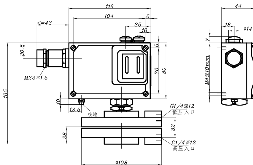
(板式安装)
