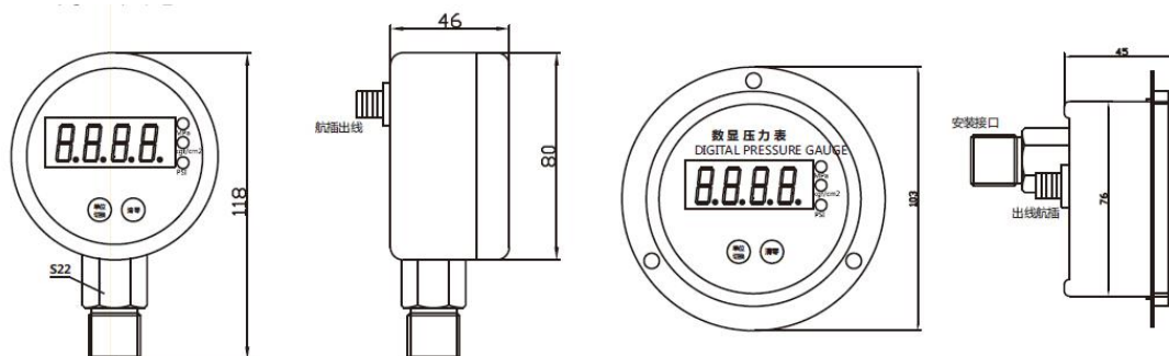
80MM 表盘
