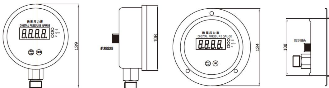
100MM 表盘
